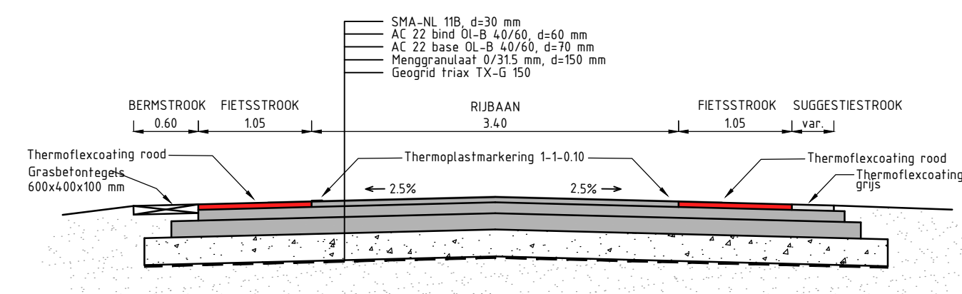
PRINCIPEDOORSNEDE (schaal 1:50)
